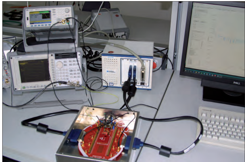
Versuchsaufbau im Bereich der Mikroelektronik
